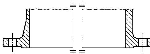
Typ 21 Integralflansch
